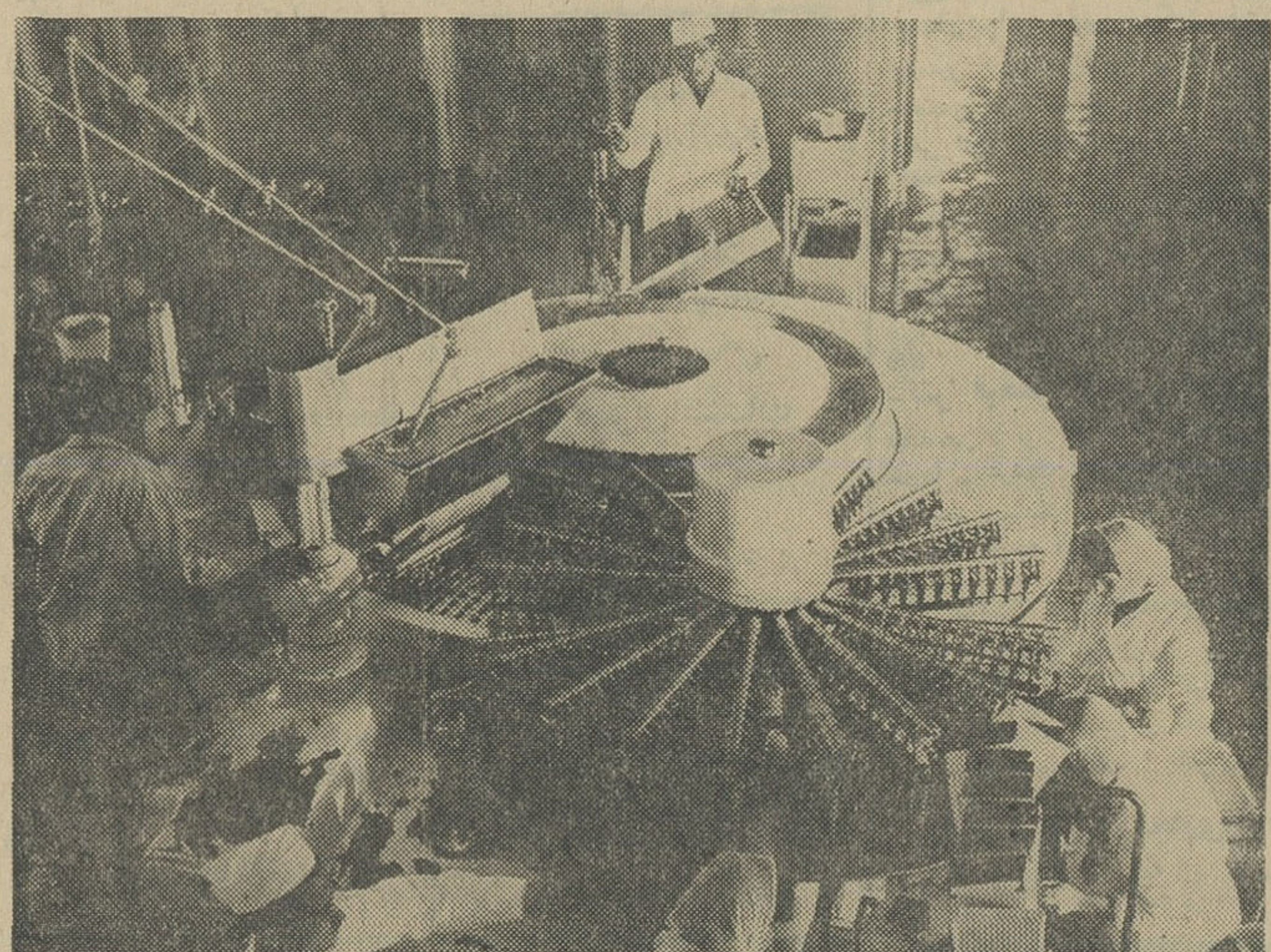
یک قسمت از دستگاه های اتوماتیک بستنی سازی کاناداداری است
